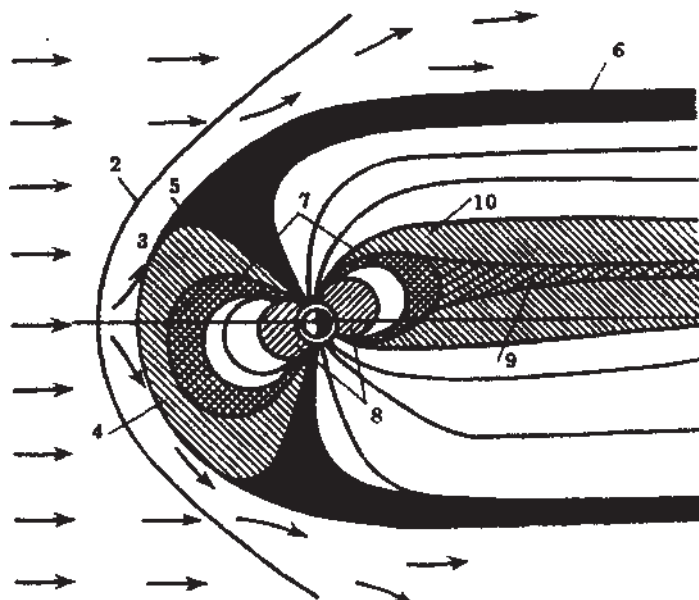
Рисунок 2.5 — Меридиональные сечения магнитосферы Земли: 1 — солнечный ветер; 2 — ударный фронт; 3 — магнитная полость; 4 — магнитопауза; 5 — верхняя граница магнитосферной щели; 6 — плазменная мантия; 7 — внешний радиационный пояс; 8 — внутренний радиационный пояс или плазмосфера; 9 — нейтральный слой; 10 — плазменный слой.
