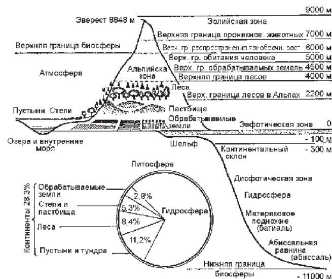
Рисунок 15.60 — Протяженность биосферы по вертикали и соотношение поверхностей, занятых основными структурными единицами (по Ф. Рамаду, 1981)
