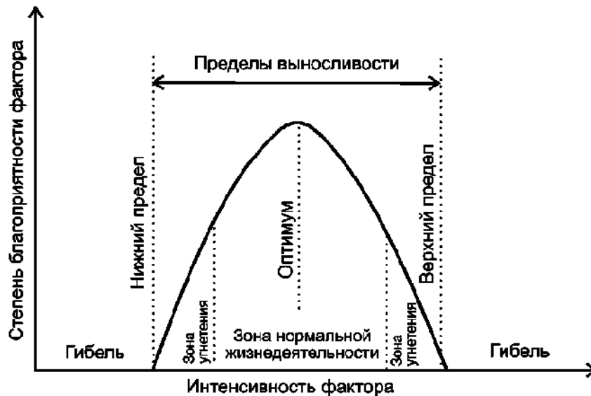
Рисунок 3.1 — Зависимость действия экологического фактора от его интенсивности
