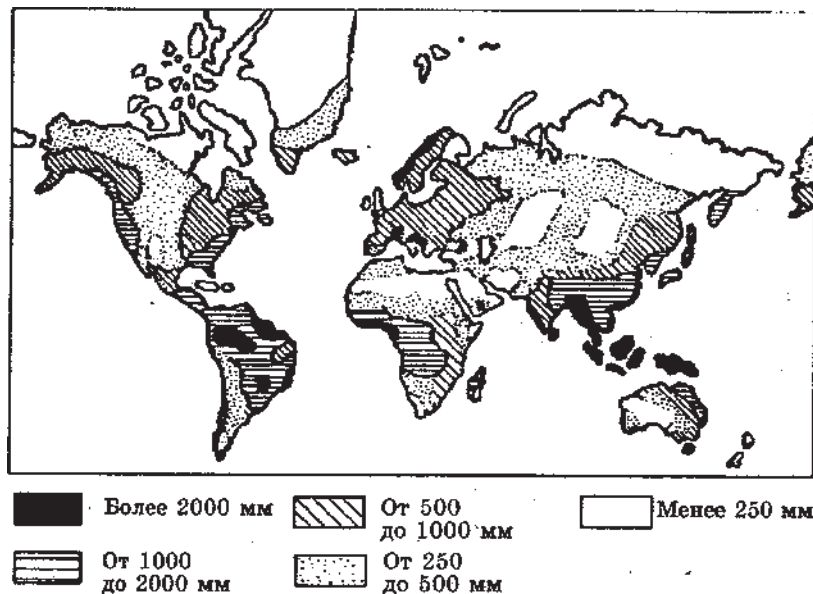
Рисунок 15.3 — Распределение годовичного количества осадков по земному шару
